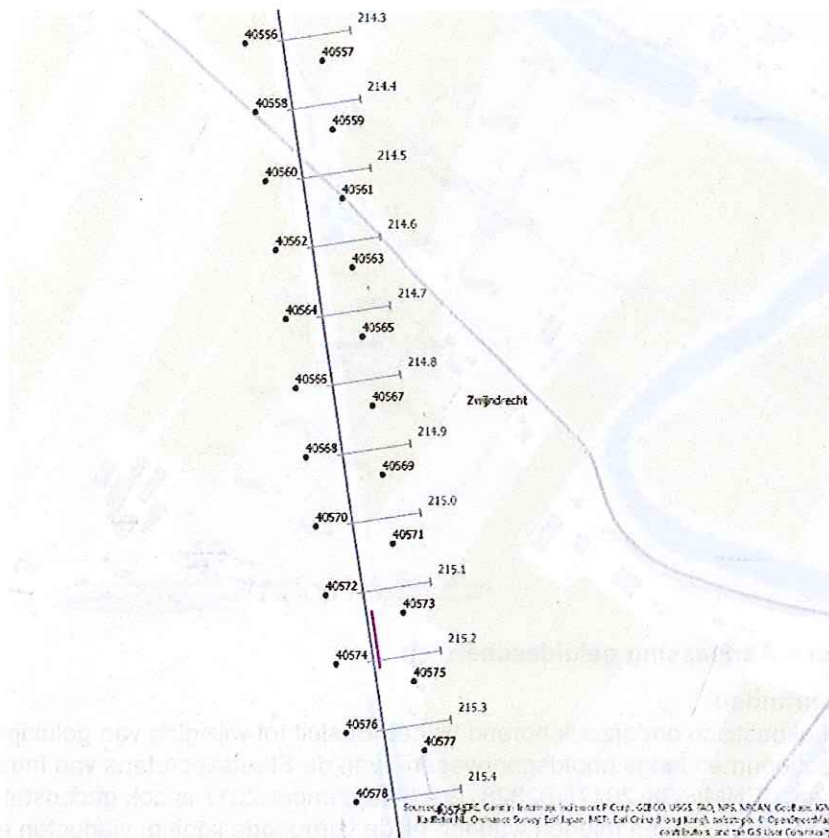
Figuur 3 Aanpassing geluidsscherm
