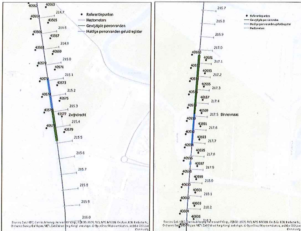
Figuur 5 Toegevoegde perronranden rond km 215 en 217
