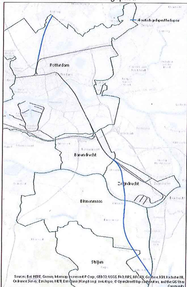
Figuur 1 Spoor waar gerekend is met akoestisch geslepen Rhedaspoor
