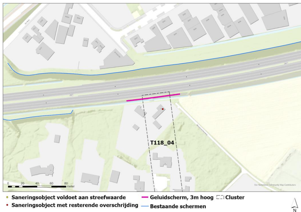
Figuur 3-1 Geluidbeperkende maatregel gemeente Veldhoven
